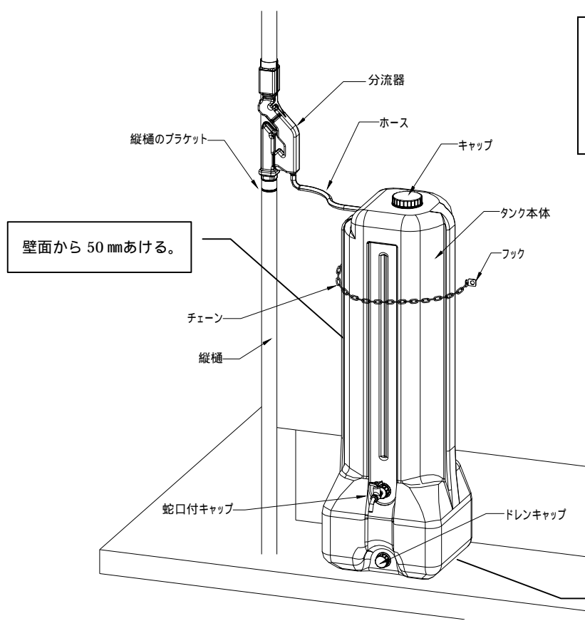
《施工完成図》
