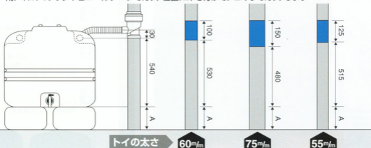
カット位置と寸法 (mm)
